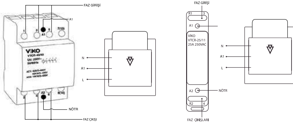
Energy Saver Mekanik Anahtarlı 230V Bağlantı Şeması
